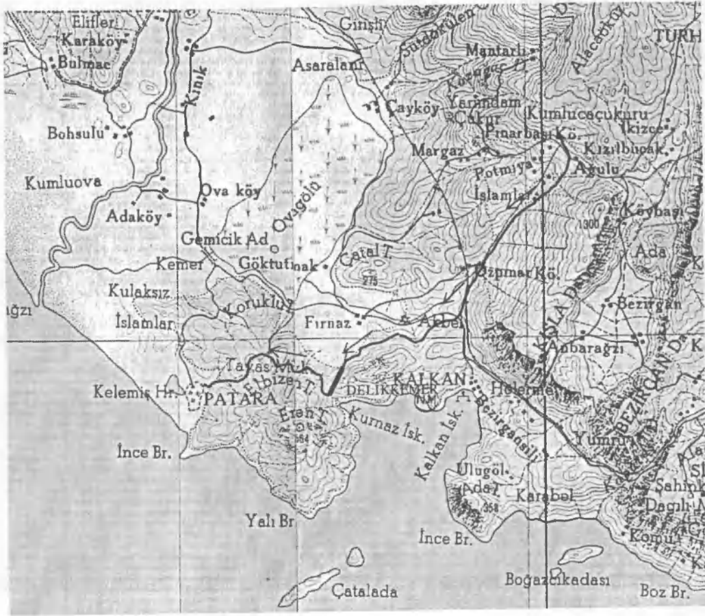
Abb. 18 Wasserleitung von Patara und Druckrohrquädukt bei Delikkemer (Ausschnitt aus der Türkei-Karte 1:200000, Blatt Keleşmiş 29-30 II ğ)
