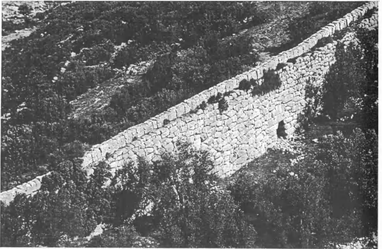
Abb. 21 Delikkemer von Osten aus der Luft
