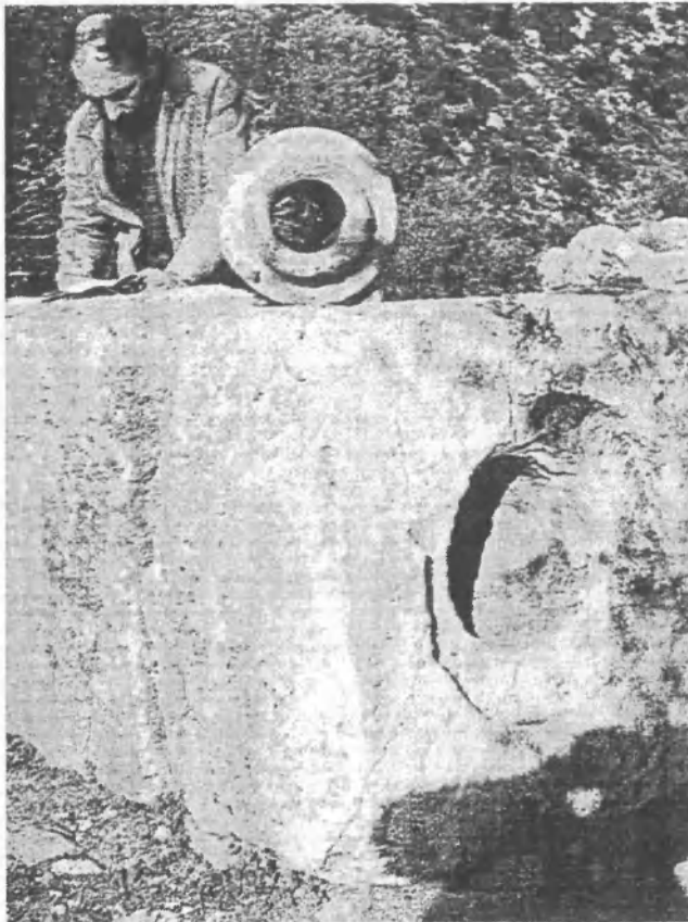
Abb. 32 Tonrohr im Vergleich mit dem Steinrohr (Foto: G. Büyükyıldırım)
